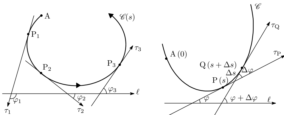
Figure 1.5: 曲率の定義と変化
