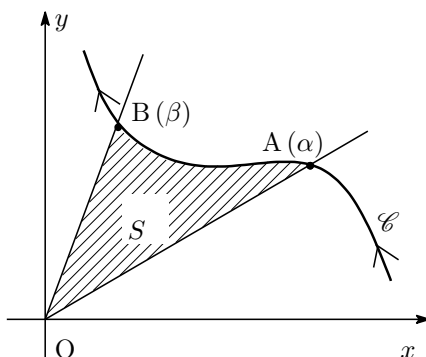
Figure 2.2: 広義の扇形
